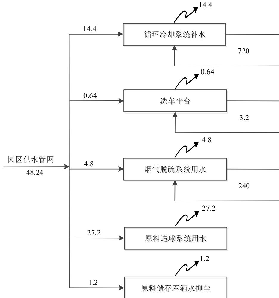
图1 本项目运营期非采暖期用排水平衡图 单位m 3 /d
