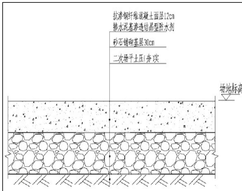
图 7 本项目一般污染区防渗结构示意图
