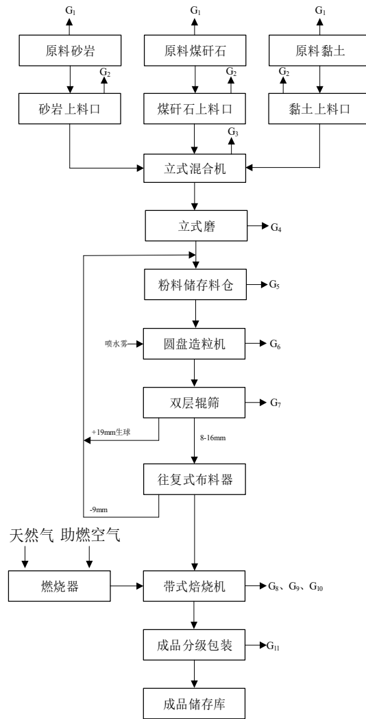
图4 本项目运营期陶粒中试线生产工艺流程及产排污环节图
