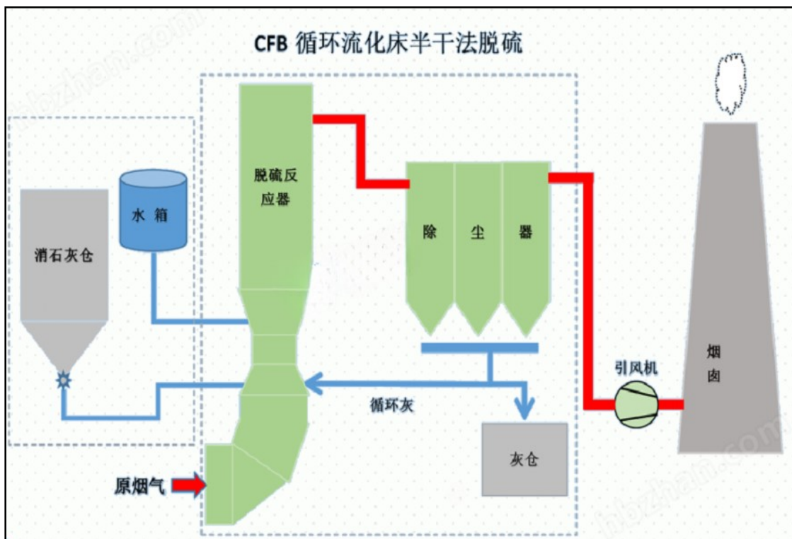
图5 CFB 循环流化床半干法脱硫技术工艺流程图
