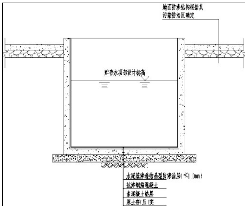
图 6 本项目重点防渗区地面防渗结构示意图
