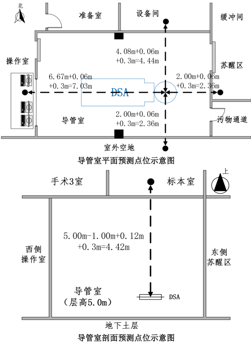
图 11-1 导管室预测点位示意图
