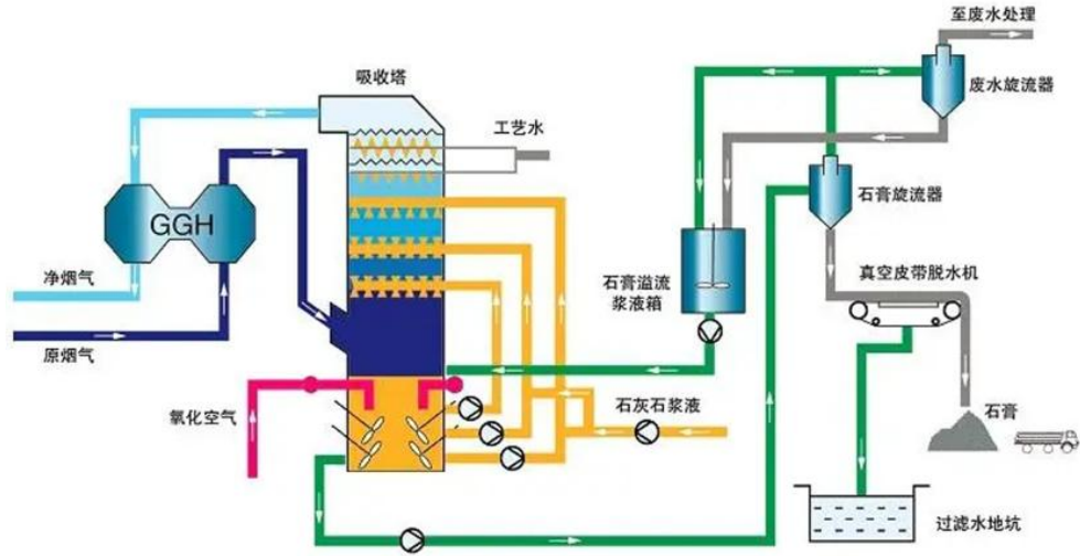
图 4.1-1 石灰-石膏法脱硫工艺流程图
