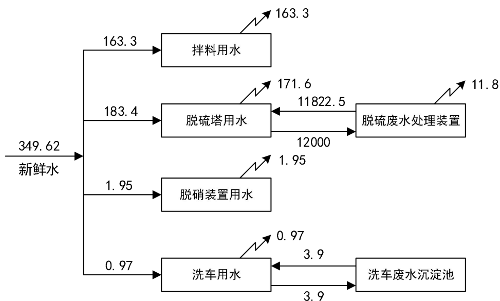
图 2.7-1 本次技改扩建项目新增用排水平衡图 m 3 /d
