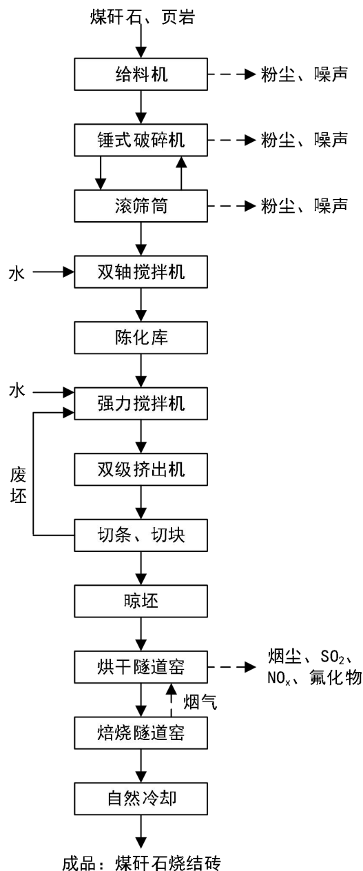
图 2.8-1 运营期工艺流程及产排污环节示意图
