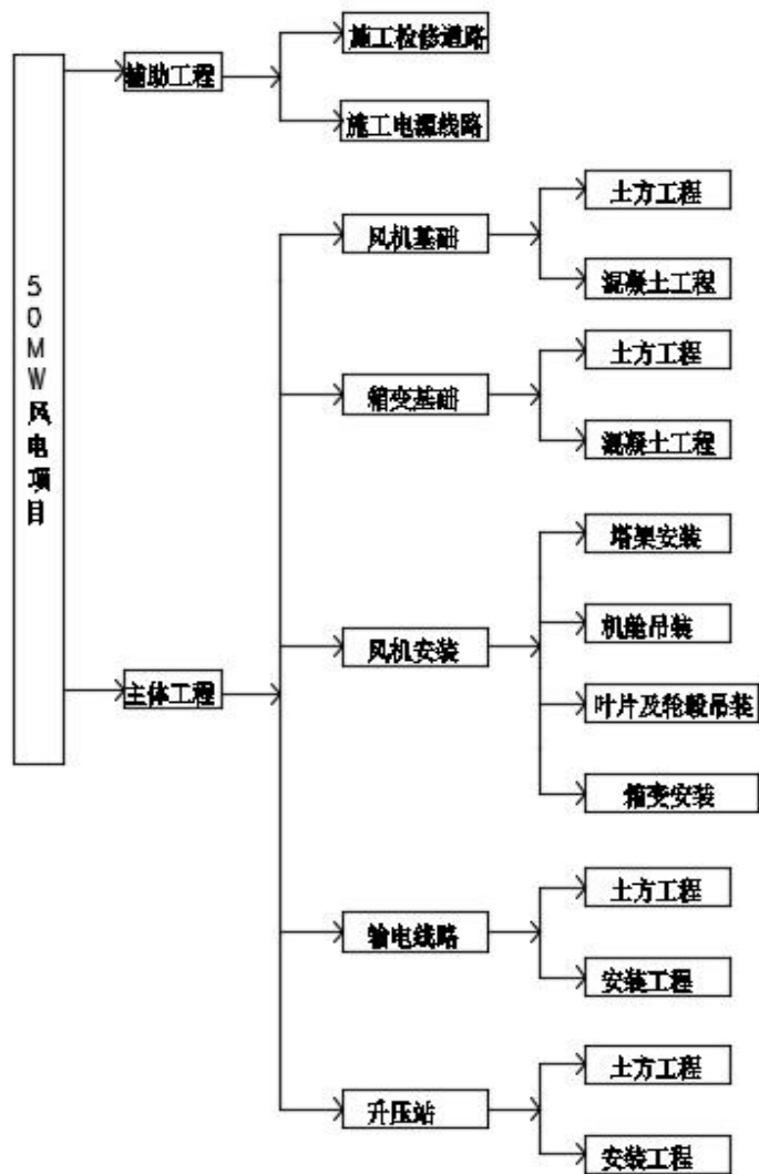
图 2-1 施工工艺图
