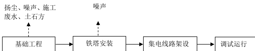
图 2-1 施工工艺图
