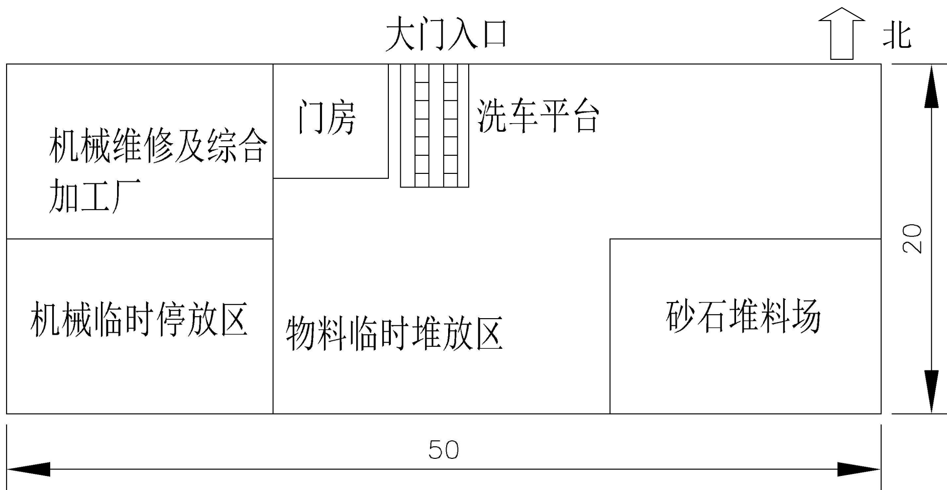
附图 6 施工临建区平面布置图
