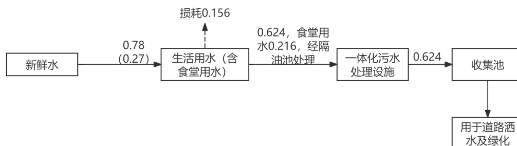
图 2-2 本项目采暖期水平衡图 单位 m 3 /d
