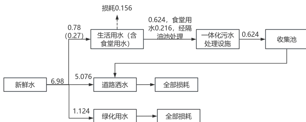
图 2-2 本项目非采暖期水平衡图 单位 \text{m}^3/\text{d}
