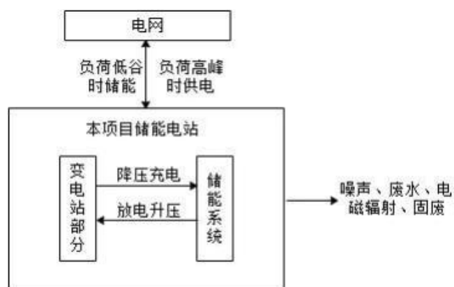
图 2-3 生产工艺及污染流程图
