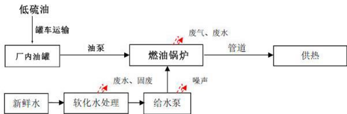
图 6 本项目锅炉运营期工艺流程及排污情况示意图
