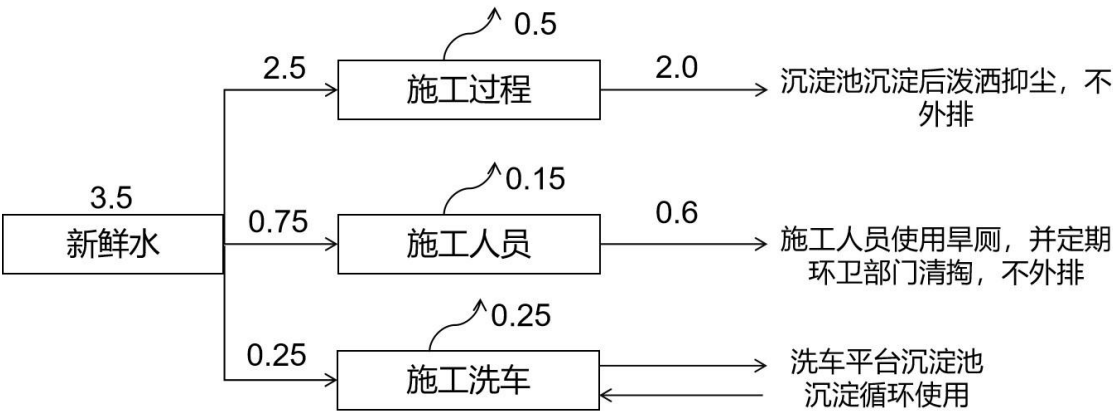
图 1 本项目建设施工期水平衡图 (m³/d)
