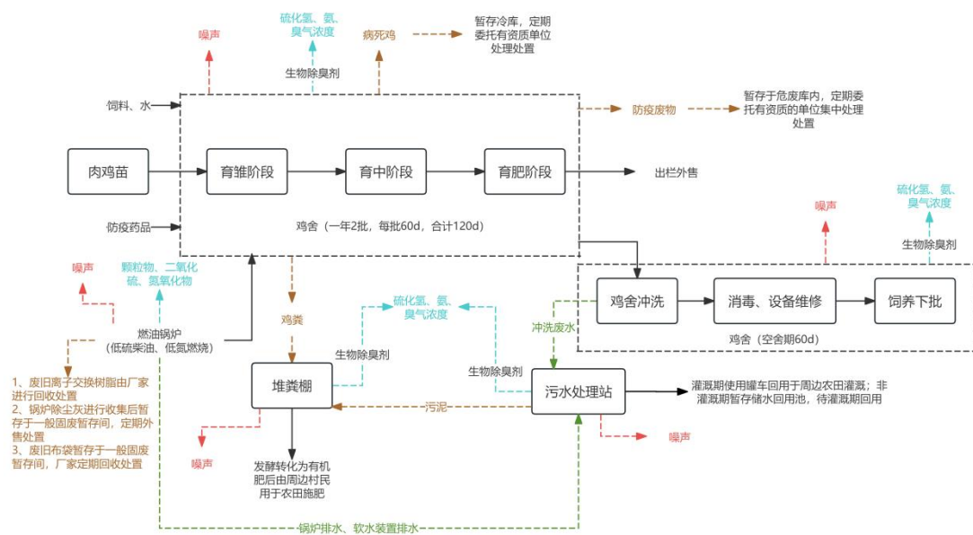
图 4 本项目运营期工艺流程及产污环节示意图
