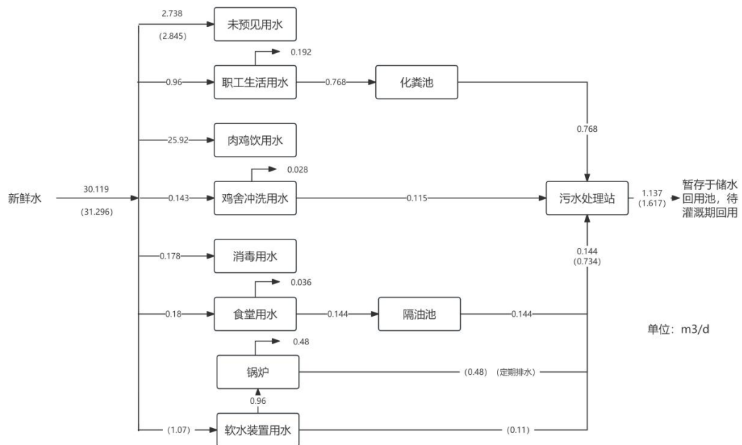
图2 本项目运营期水平衡图 (m³/d)
