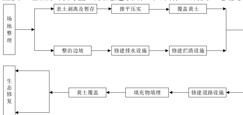
图 3-9 本项目填充及生态修复作业流程图
