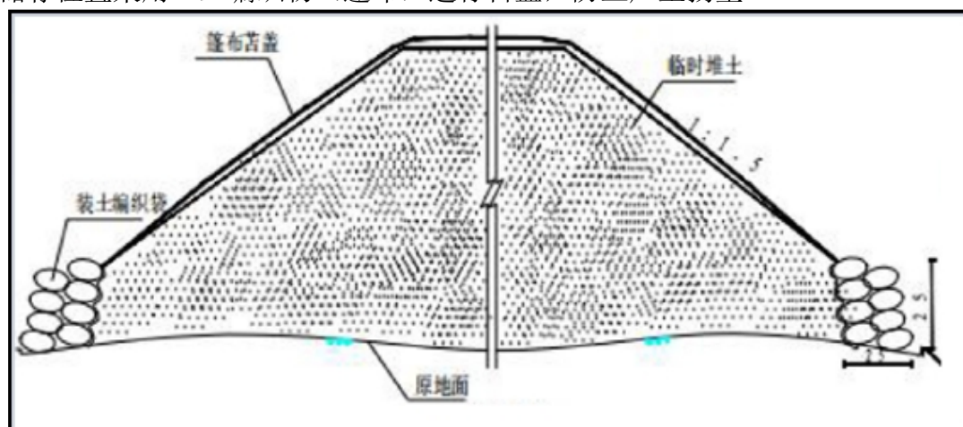
图 3-10 本项目临时堆土防护措施示意图
