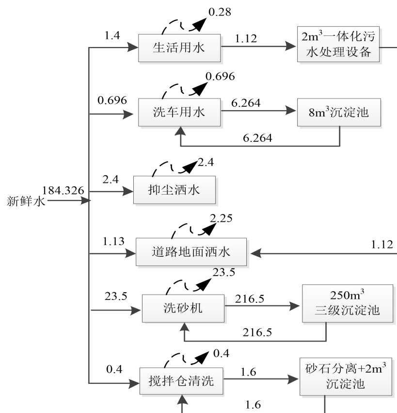
图 2.7-1 项目水平衡图 (单位: m³/d)
