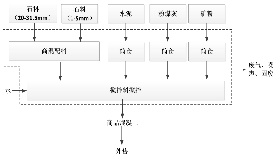
图 2.8-4 商混工艺流程及产排污物节点图
