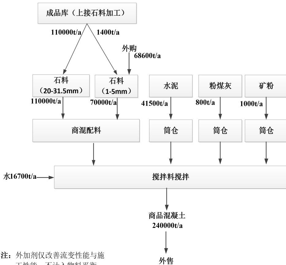
图 2.4-3 商混物料流向图
