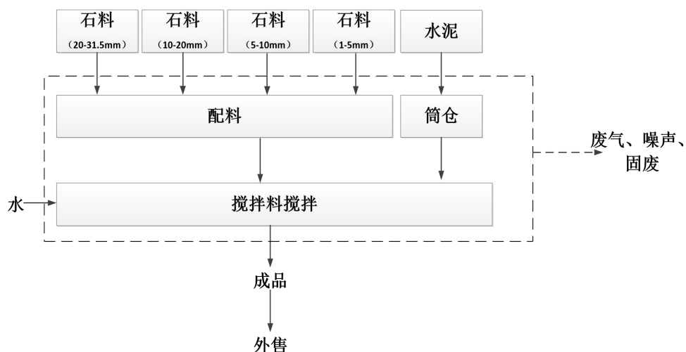
图 2.8-3 水稳料工艺流程及产排污物节点图
