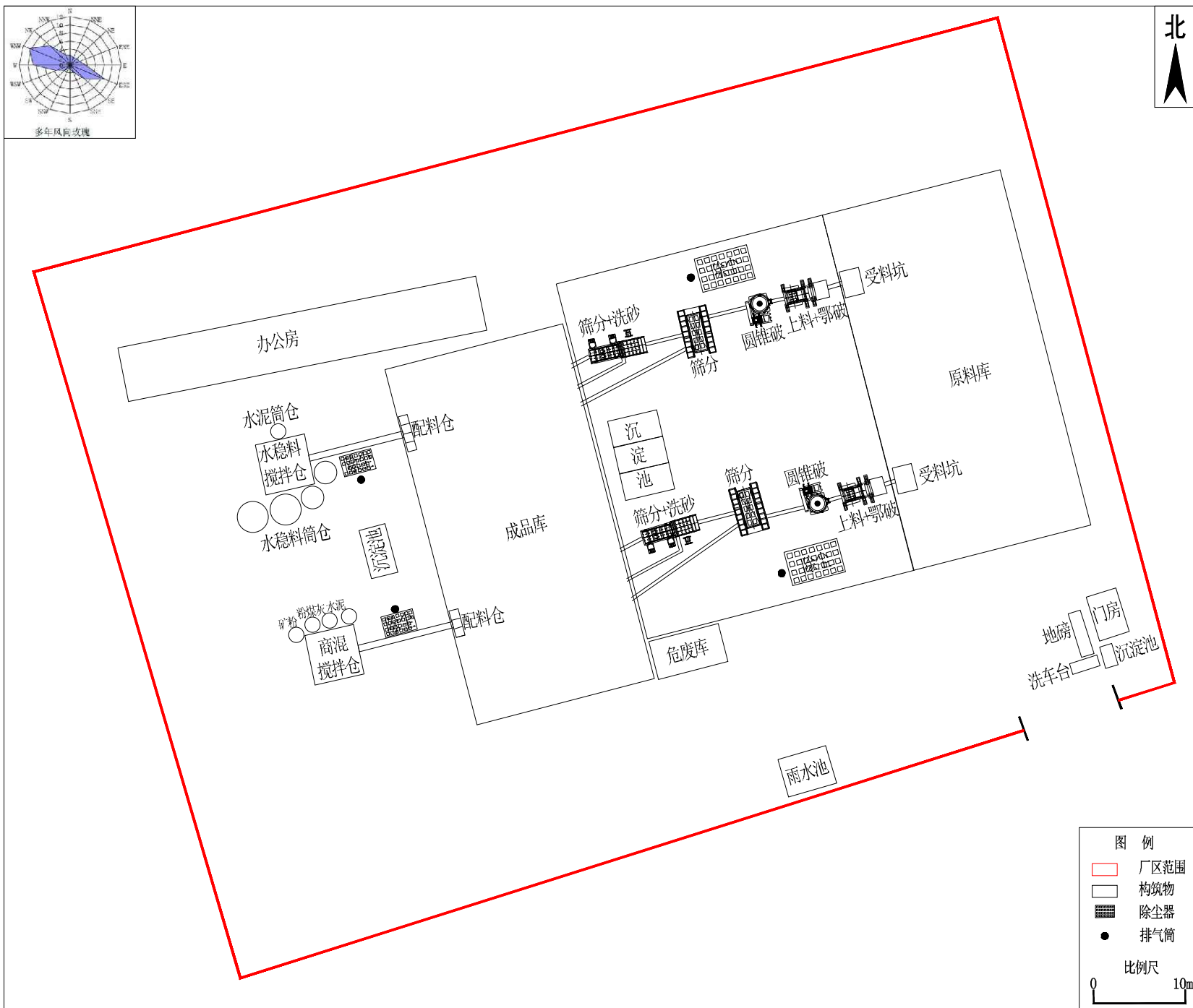
附图2 项目总平面布置图
