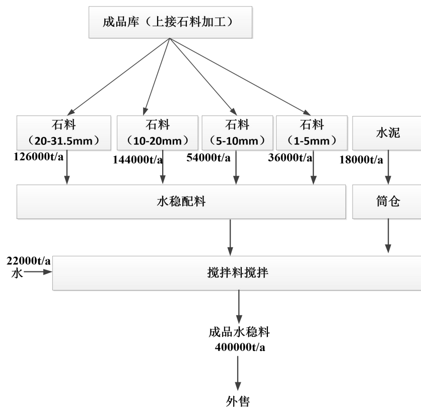
图 2.4-2 水稳料物料流向图
