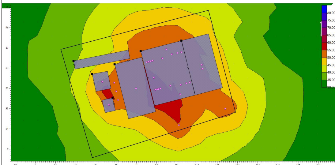
图 4.8-1 厂界噪声预测等声级线图
